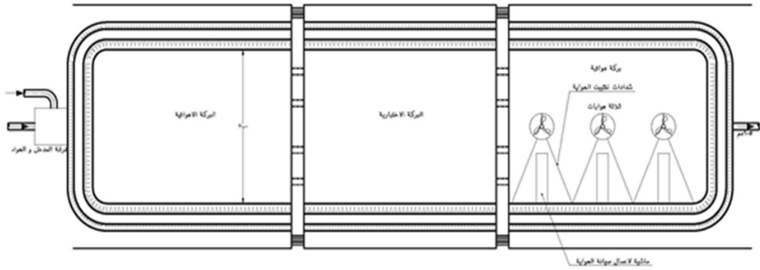
شكل تخطيطي لنظام المعالجة باستخدام برك الأكسدة المتهواة ميكانيكيا
