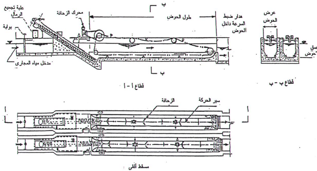
شكل رقم (٣) تفاصيل أحواض فصل الرمال
