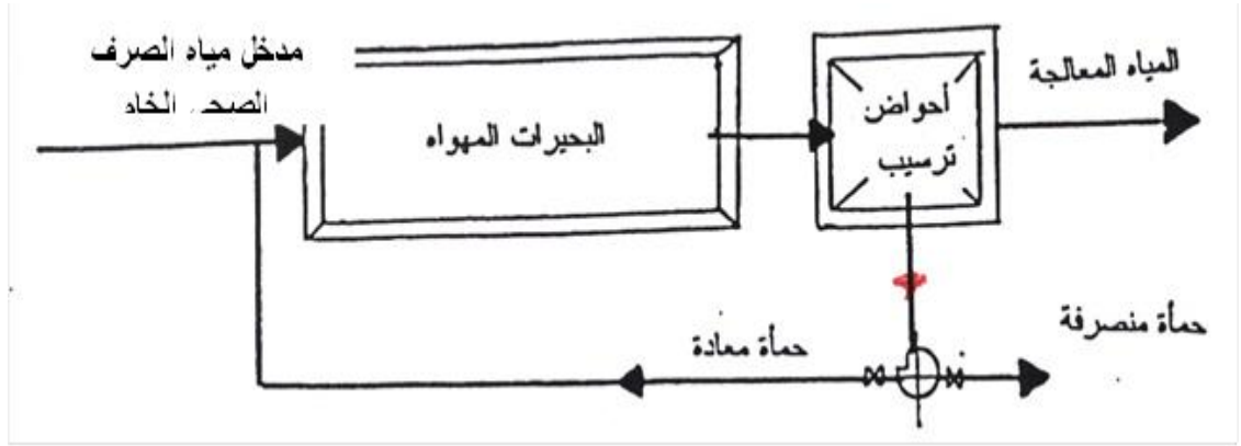
شكل رقم (١٤-٢) مسار مياه الصرف الصحي في البحيرات المهواة (تهوية ممتدة)
